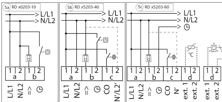
Huonetermostaatin kytkentä
